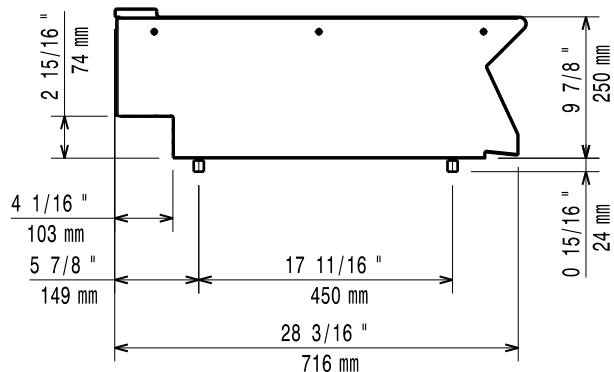
Felülnézet
